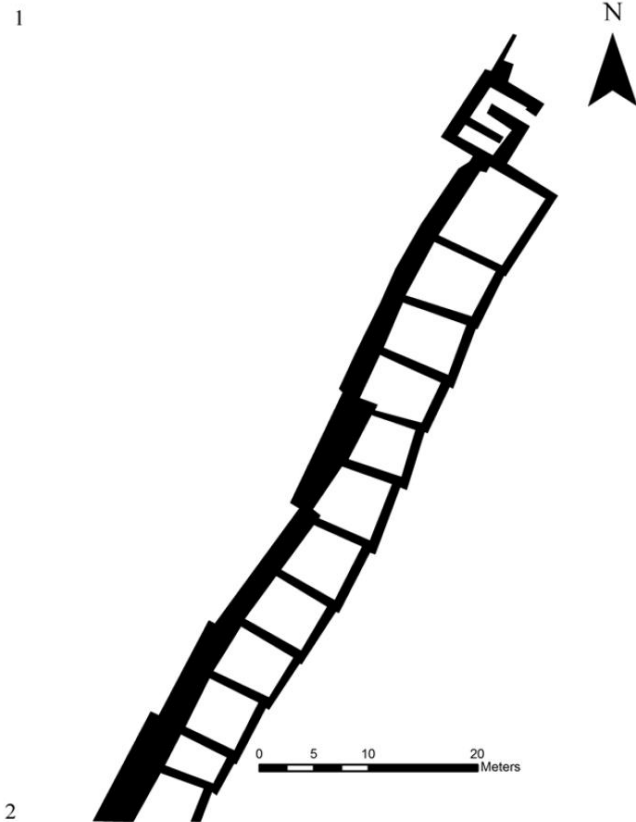
Figure 6.7 Defenses at Alişar: 1 Postern gate (after von der Osten 1937: fig. 29). 2 Casemate wall (after von der Osten 1937: fig. 24)
